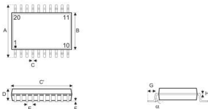
20-pin SSOP(150mil) 外形尺寸
